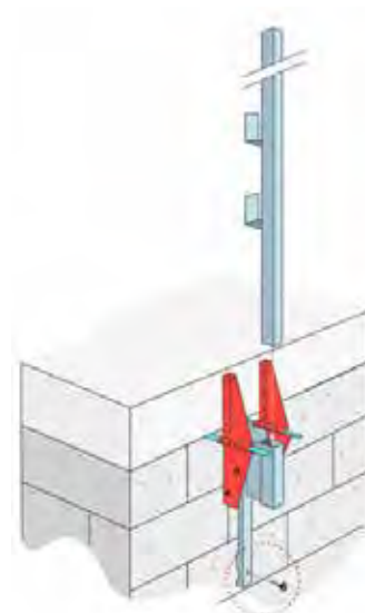
Protection périphérique après coulage de la dalle Rand bescherming na het realiseren van de betonplaat.
