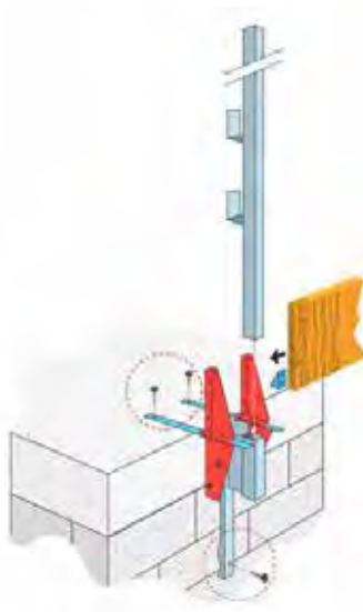
Protection périphérique sur dalle existante Rand bescherming op de reeds bestaande betonplaat
