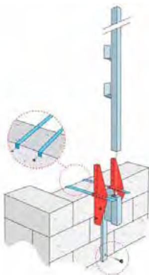
Protection périphérique avant réalisation de la dalle Rand bescherming voor het maken van de betonplaat
